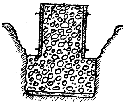
b- Fondation en béton cylopéen
