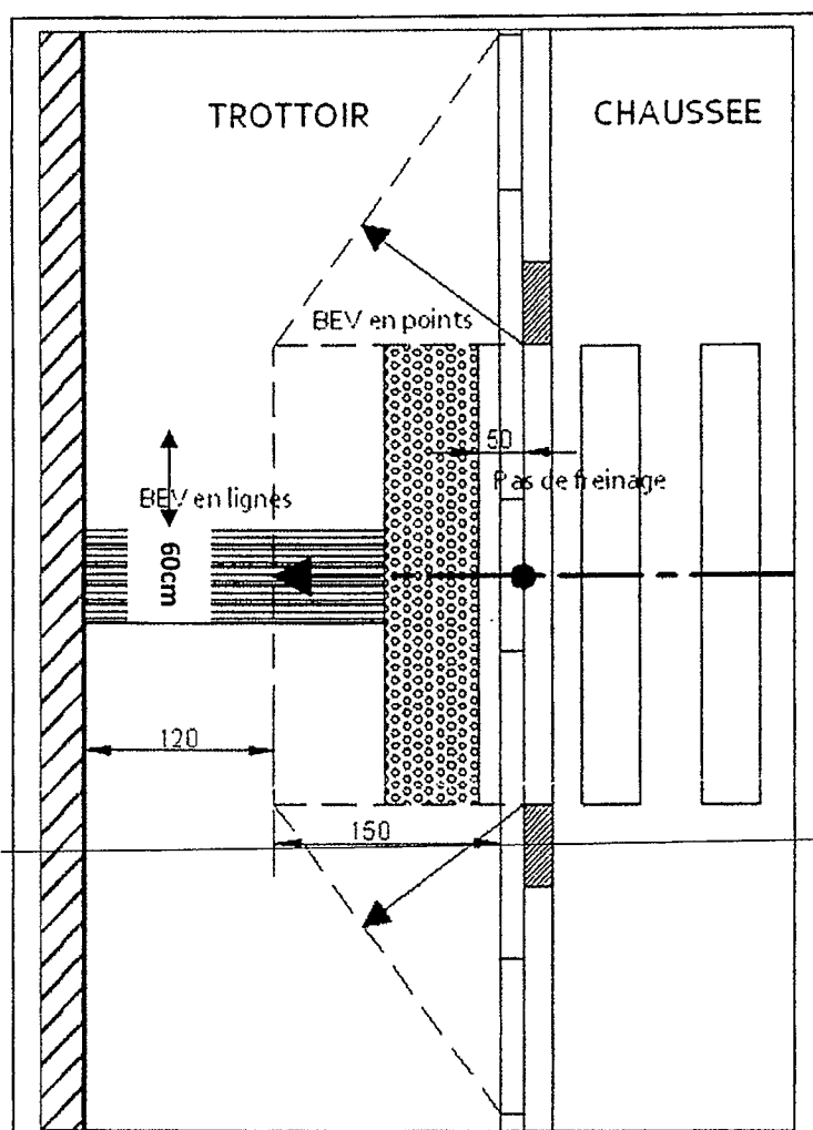
Figure 23 : bande d'éveil et de vigilance.
