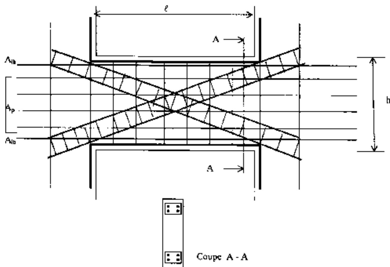
Figure 7.9 : Ferrailage du Linteau
