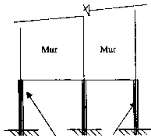
Figure 7.7 : Poteaux confinés sur toute la hauteur
