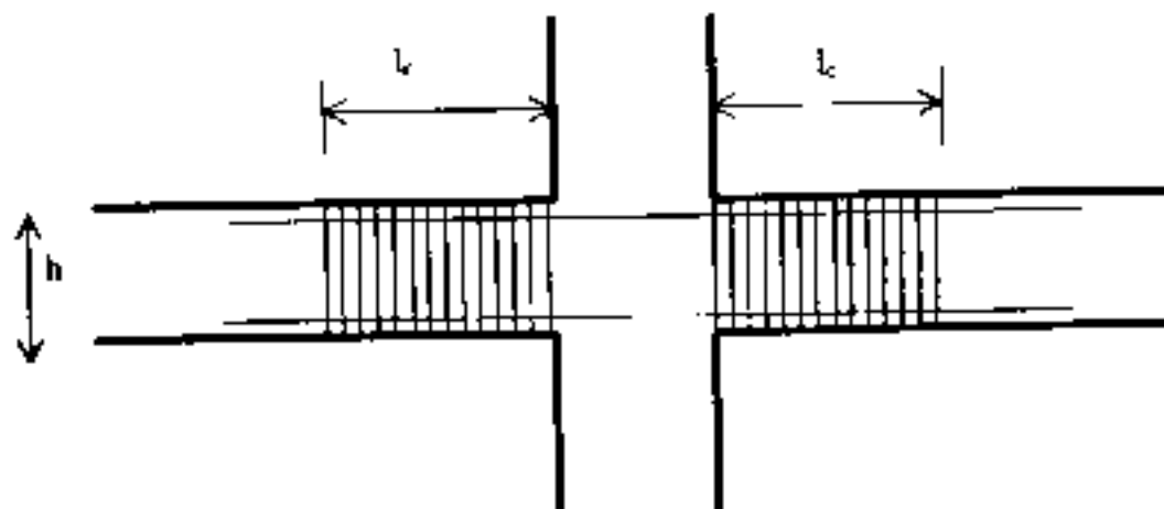
Figure 7.4 : zones critiques d'une poutre
