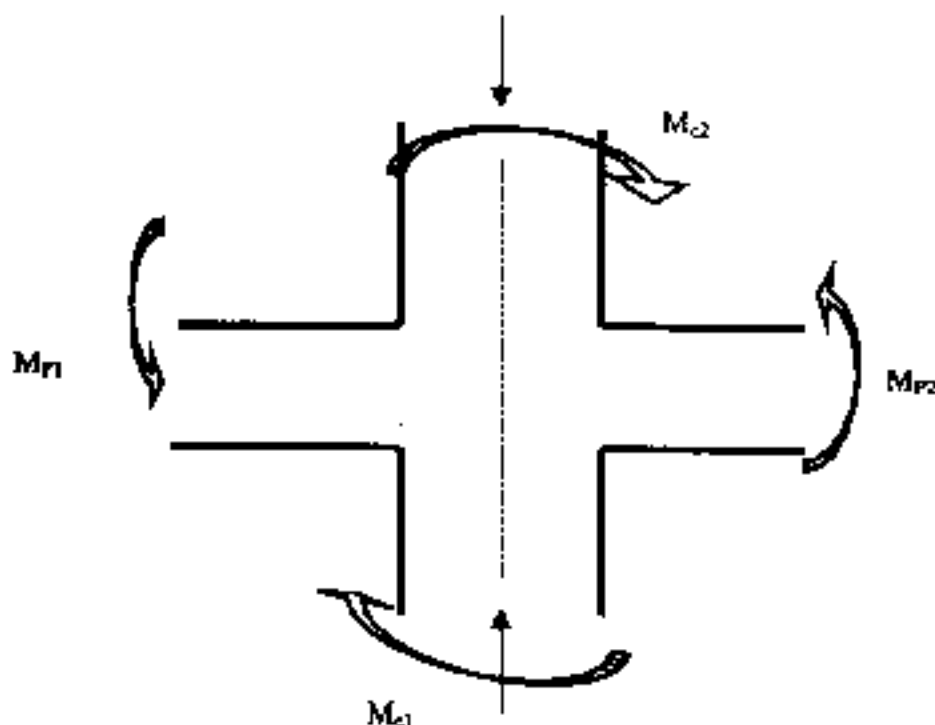
Figure 7.7 : Moments au nœud
