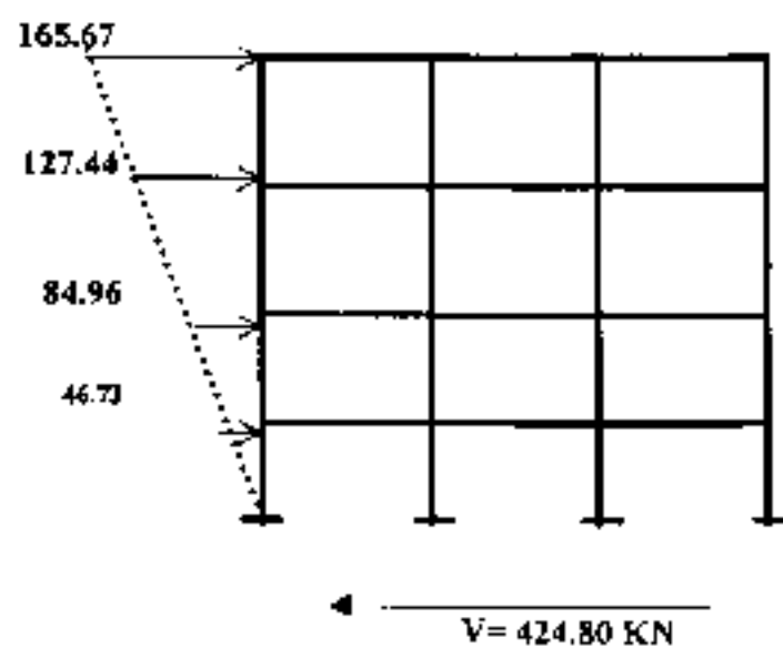
Fig. 2 Répartition de la force sismique V
