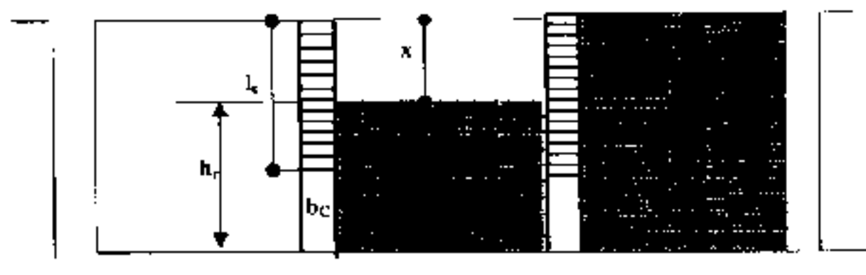
Figure 7.6 : zone critique poteau-remplissage
