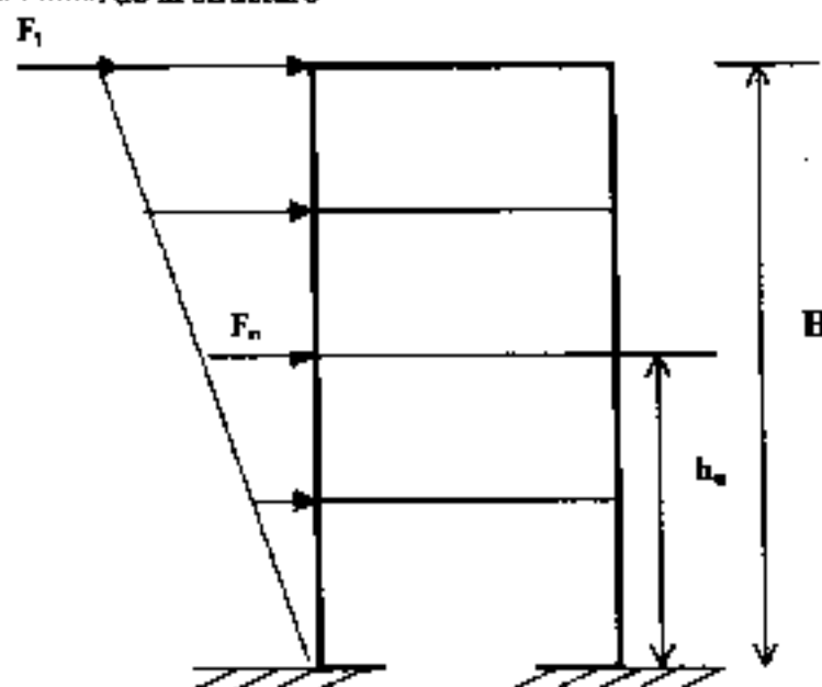
Figure 6.1 : Répartition verticale des forces sismiques
