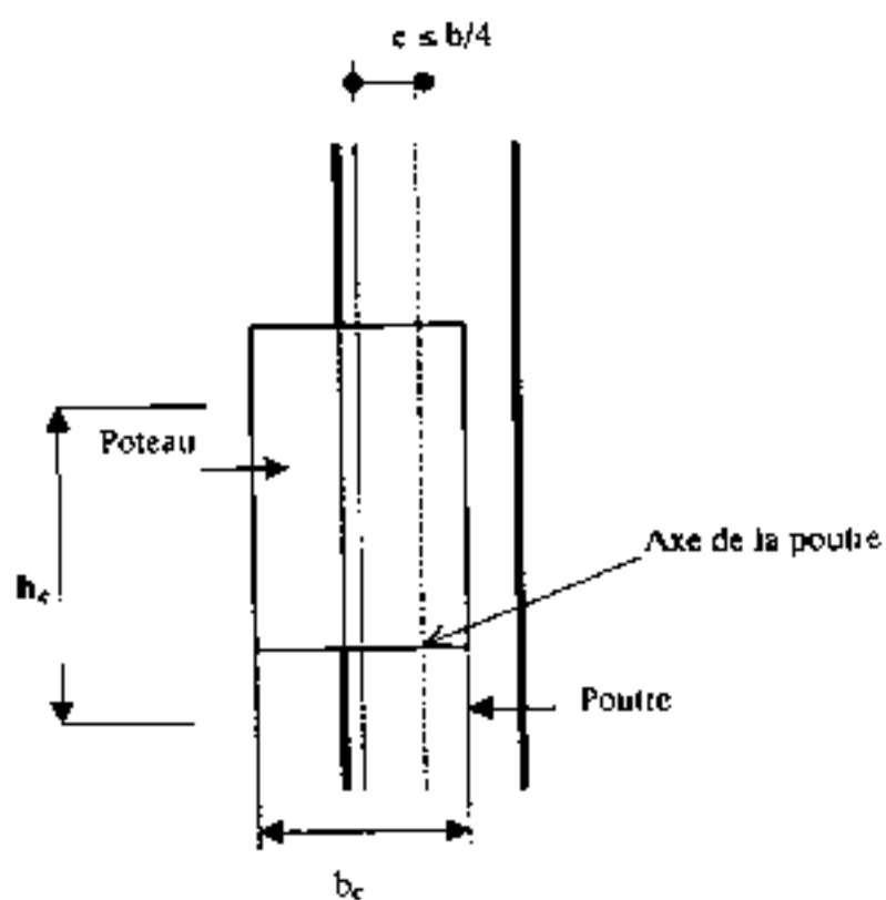
Figure 7.3 : Excentricité des axes poteau-poutre
